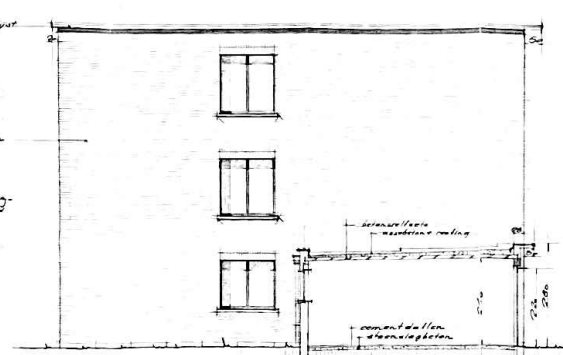
ZIJGEVEL
