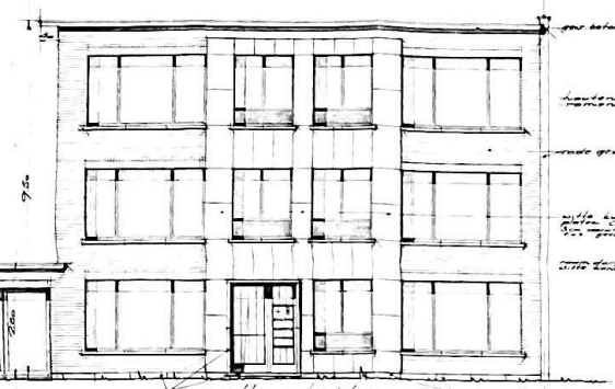
VOORGEVEL
